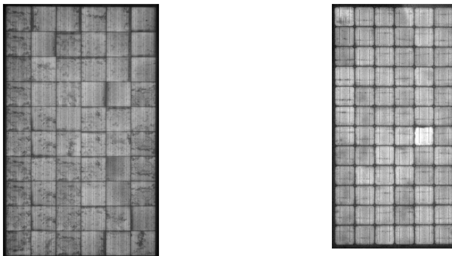
Figura 4 - Imagens de eletroluminescência de módulos dos sistemas estudados: à esquerda os módulos YL245P-29b; à direita módulos I-100/24.
