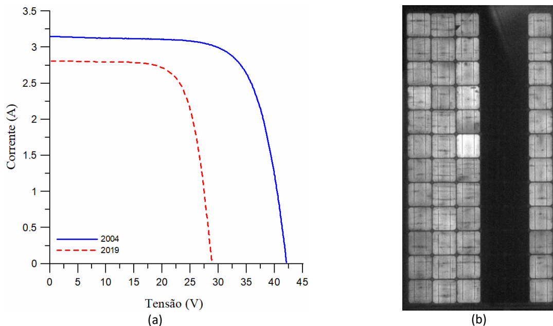
Figura 7 - (a) Curvas I-V, antes e após a instalação de um módulo do sistema de 15 anos apresentando defeitos. (a) Imagem de eletroluminescência do módulo.
