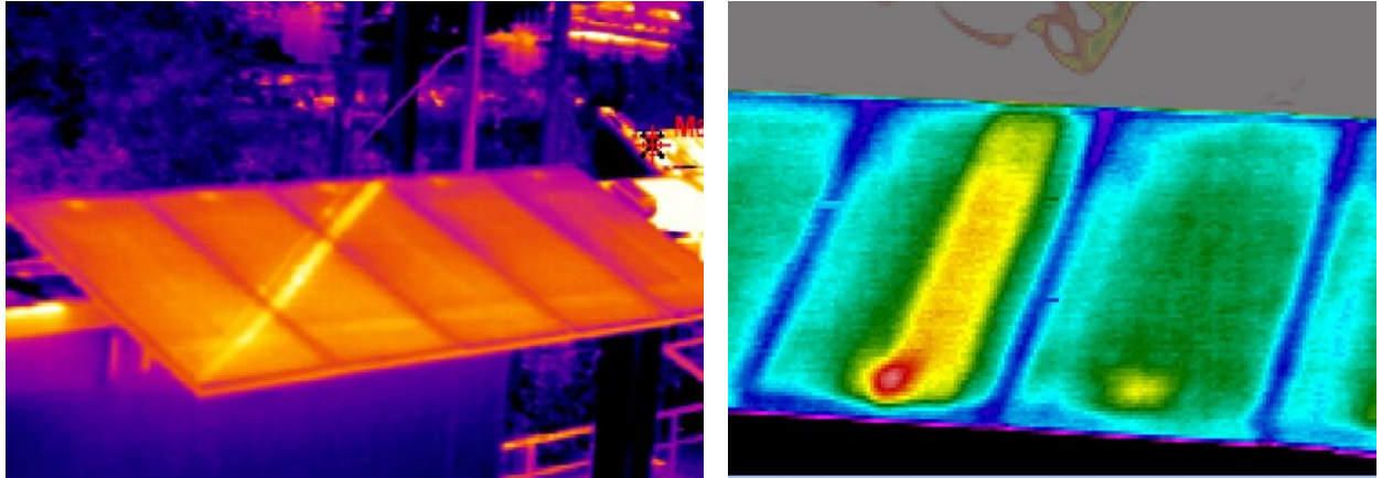
Figura 5 - Registro de imagem termográfica: à esquerda os módulos YL245P-29b; à direita módulos I-100/24.
