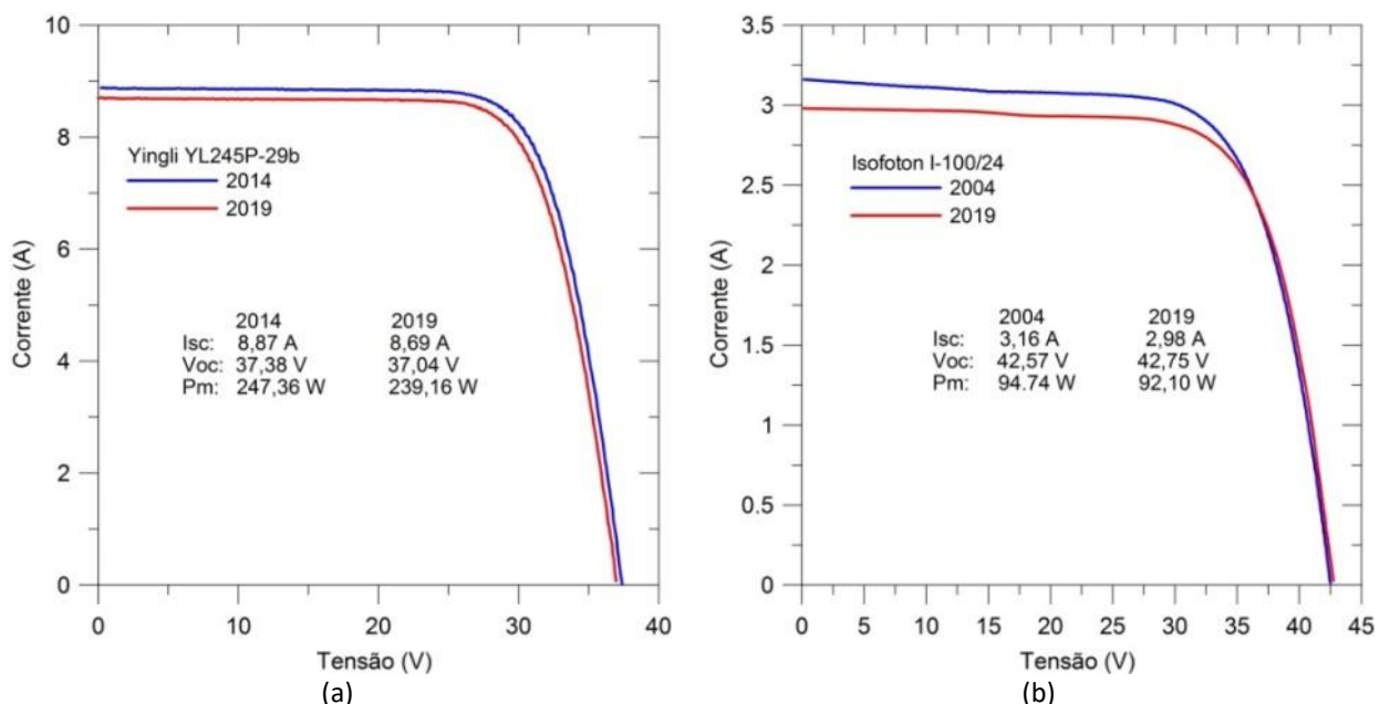
Figura 6 - Curvas I-V, antes e após a instalação, de um módulo de cada sistema sendo em (a) o modelo YL245P-29b e em (b) o modelo I-100/24.
